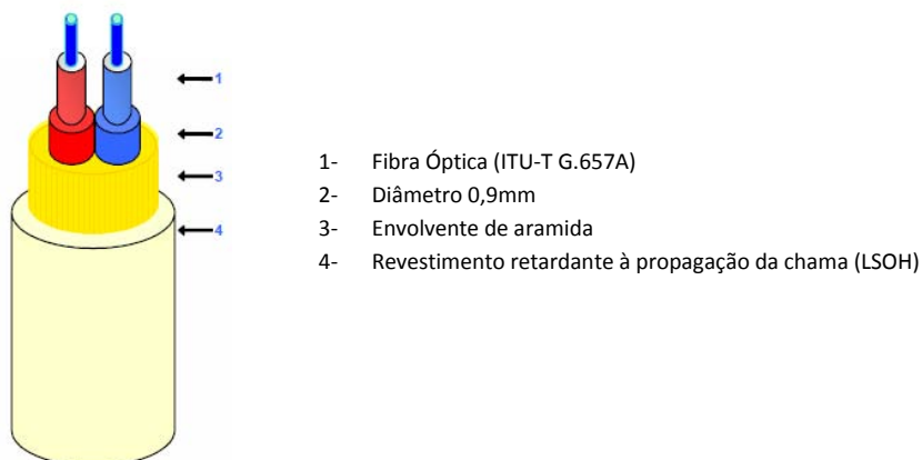
Figura 91 – Cabo individual de cliente com duas fibras
