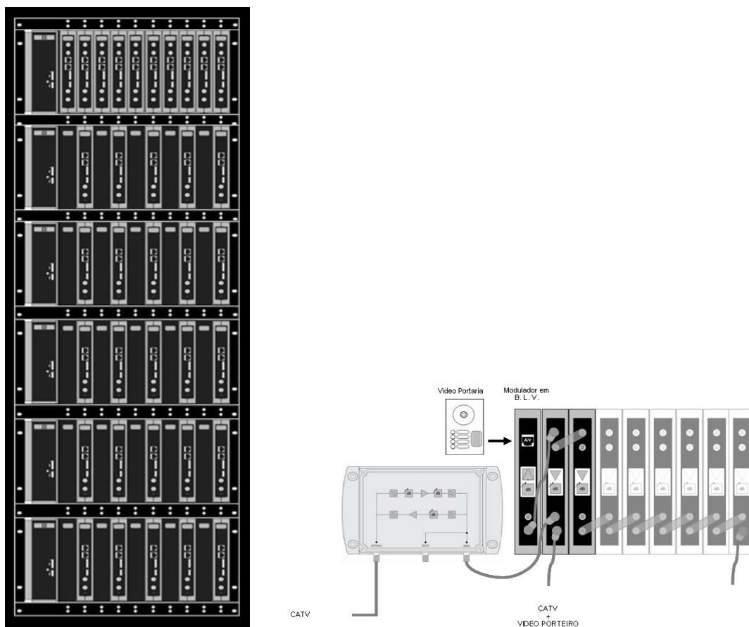
Figura 18 – CR1 e modulação de sinal de videoporteiro
