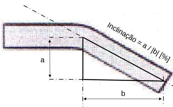
Figura 96 - Inclinação
