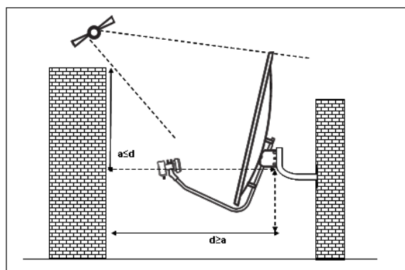
Figura 87 – Antenas parabólicas na proximidade de obstáculos
