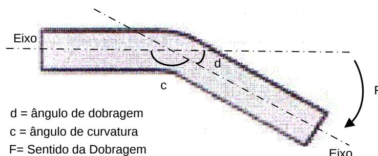
Figura 95 – Ângulos de dobragem e de curvatura
