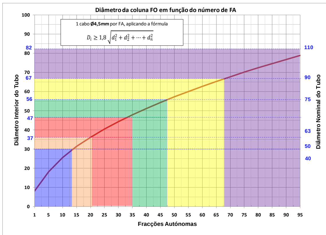
Figura 78– Diâmetro da coluna FO em função do número de FA
