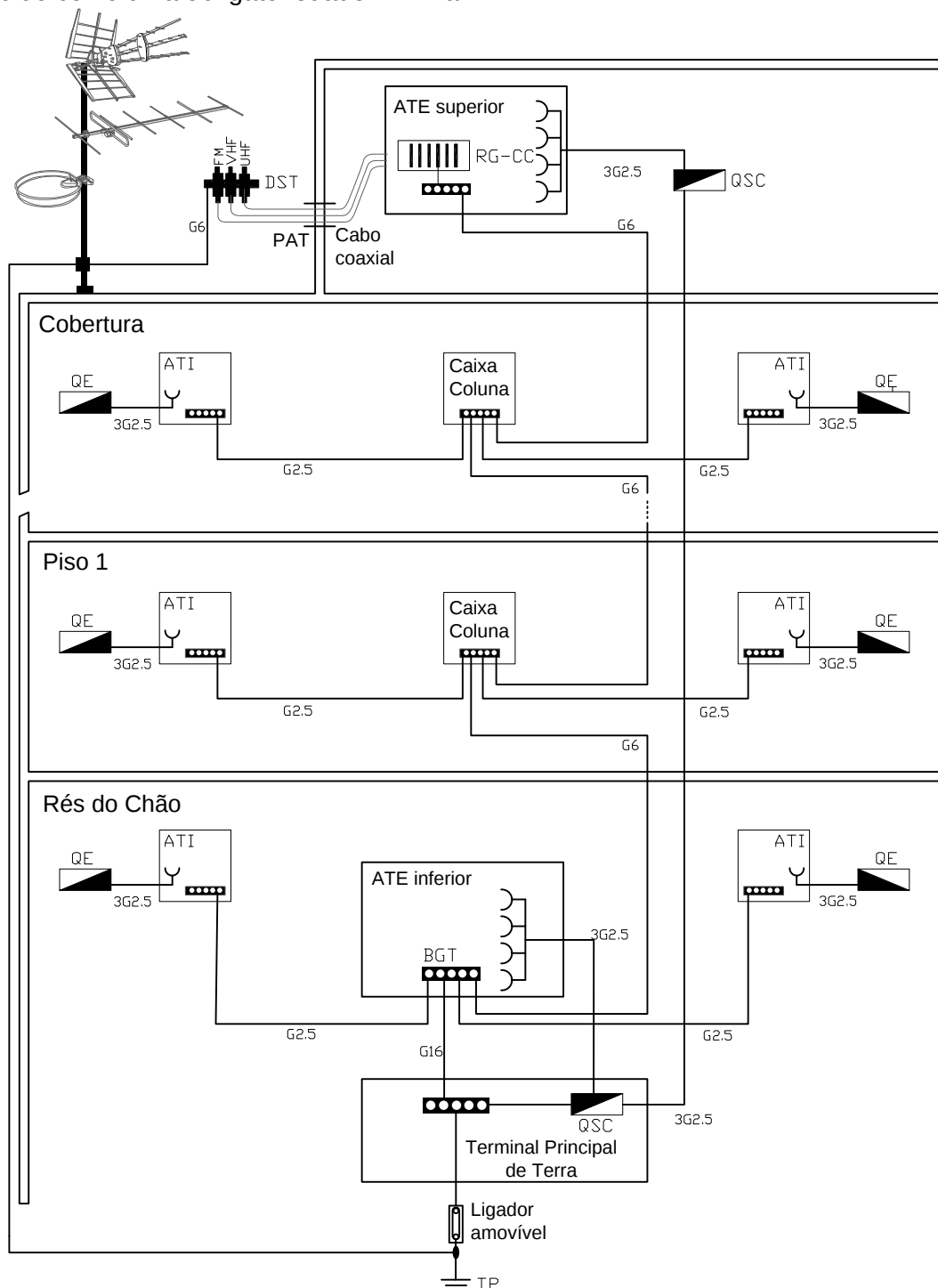
Figura 118 – Esquema eléctrico e de terras
