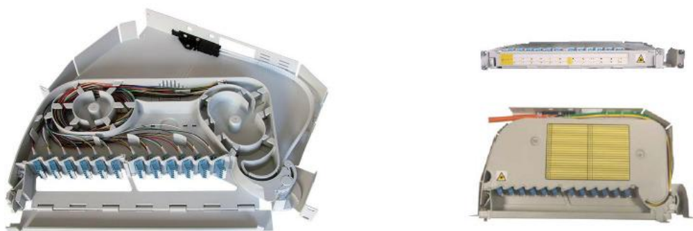
Figura 90 - Acomodação de fibras ópticas
