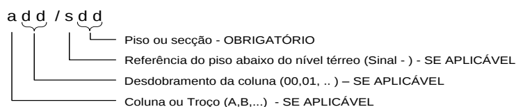
Figura 104 – Identificação das caixas da coluna montante
