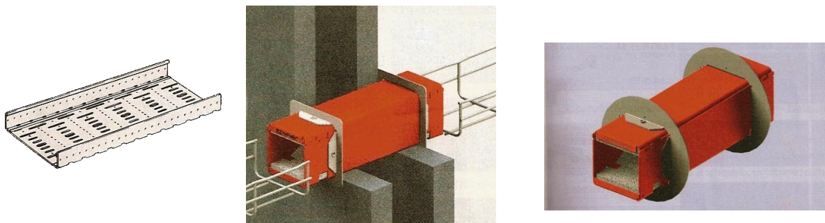
Figura 46– Esteira, atravessamento de cabos, corta-fogo para caminho de cabos
