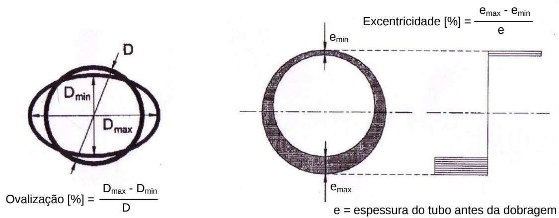
Figura 99 – Ovalização e Excentricidade
