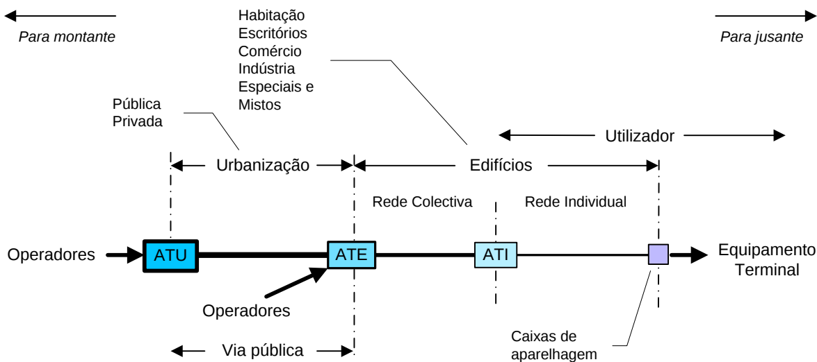
Figura 2 – Pontos de distribuição
