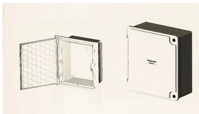
Figura 50 - Caixa para ATE e Caixa de Entrada de Moradia Unifamiliar (CEMU)
