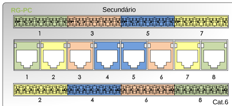
Figura 56– Unidade modular do secundário do RG-PC
