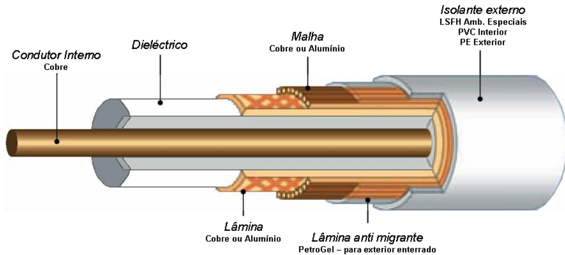
Figura 15 – Cabo coaxial
