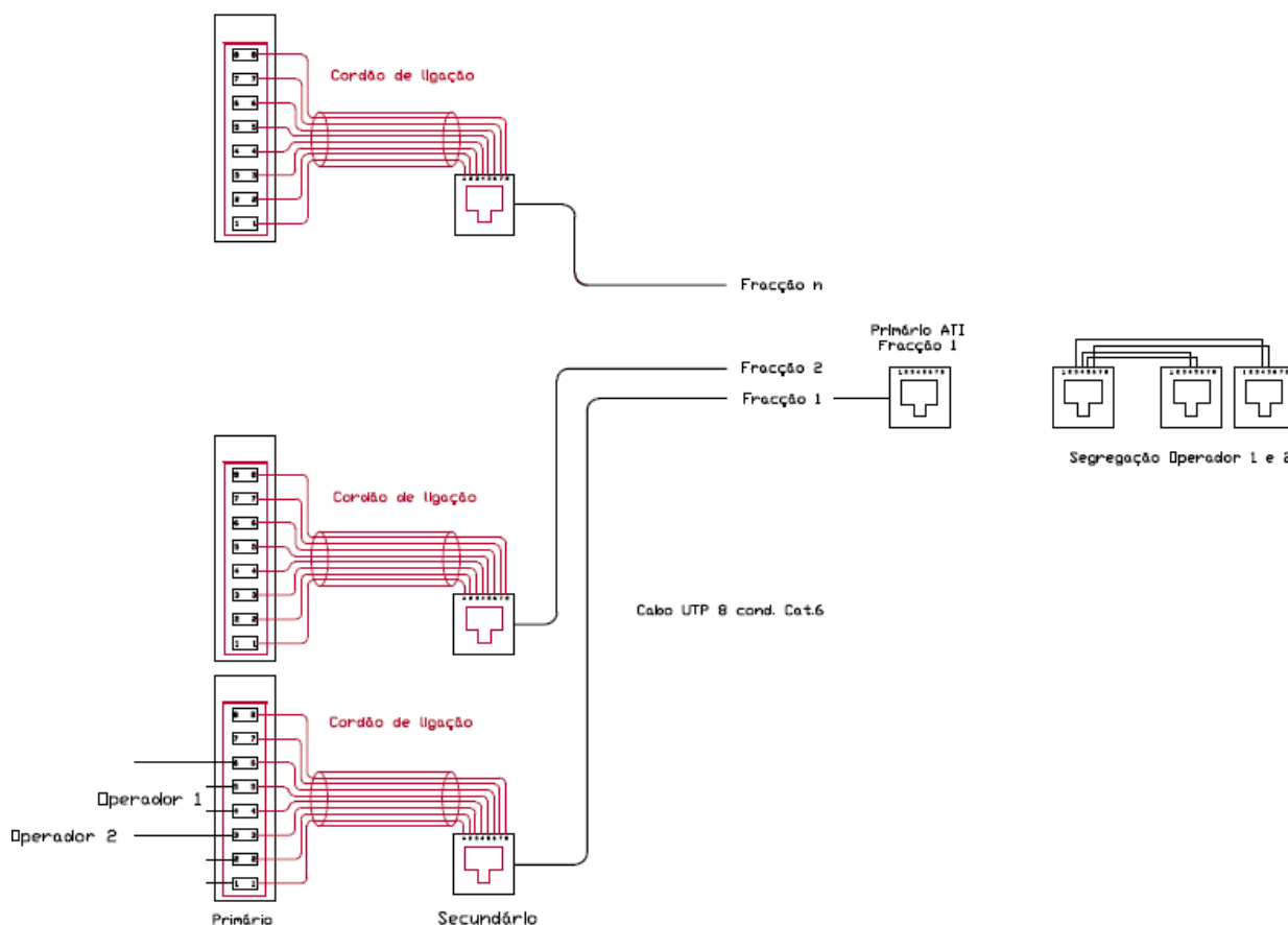
Figura 81 – Esquema exemplo de RG-PC
