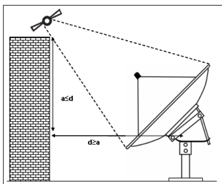
Figura 87 – Antenas parabólicas na proximidade de obstáculos
