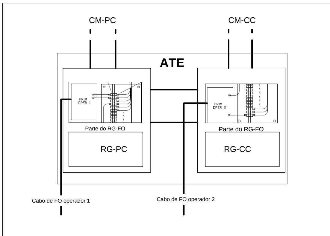
Figura 123 – Desdobramento do RG-FO nas caixas do ATE
